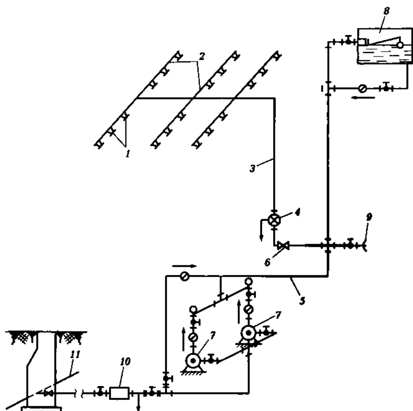
Рис. 2.5. Схема sprinkлерной установки:
